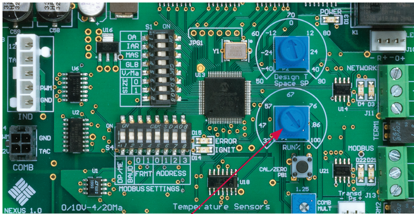
Run % Potentiometer
